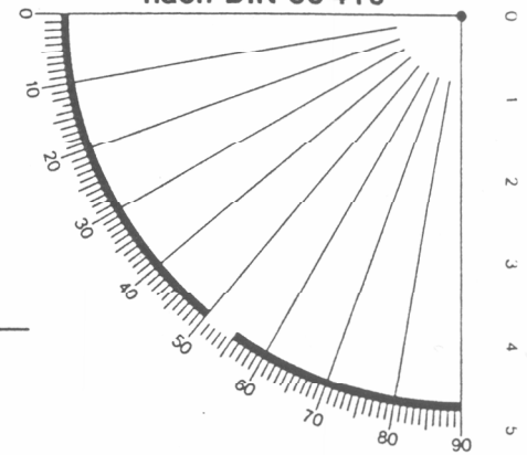
Draufsicht mit typischen Armstellungen
